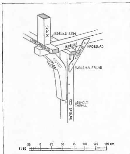
c. Samlingerne omkring gadesidens stokværksfremspring. Skråprojektion gengivet i mål 1:50.
