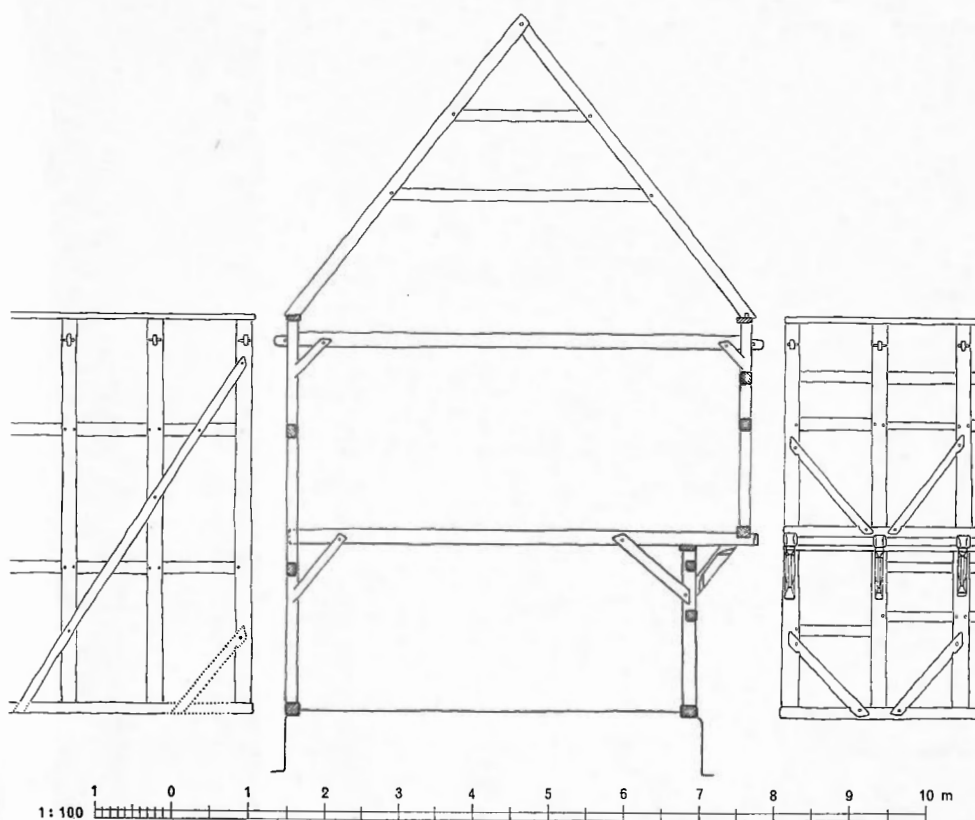
Pilegrändgården i Ystad. 11 fag lang magasinbygning opført omkr. 1490–1500 i forlængelse af et omkr. 1530 udskiftet enetages bolighus. Tværsnit med to fag af langsiden mod Pilegränd (til højre) og godt to fag af bagsiden (til venstre). Siden mod Pilegränd har korte regelmæssige anbragte skråbånd i begge etagers undertavl, medens gårdsiden er afstivet med lange udvendige ranker gående fra øverste ende af hjørnestolperne skråt ned over stolper og løsholter til fodrem midt i 3. fag fra hjørnerne. Opmåling 1:100. Tegnet af HHE.
