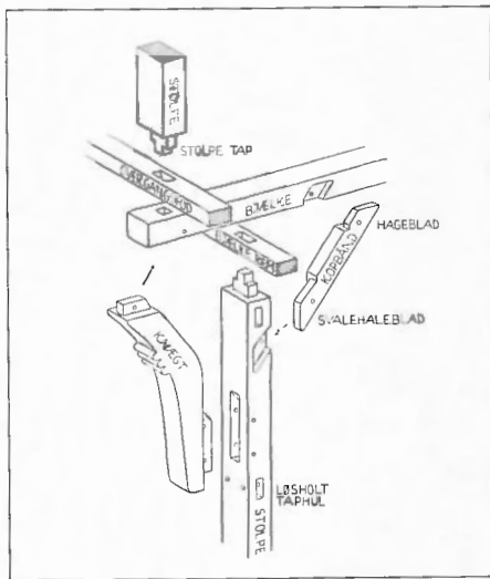
d. Samlingerne omkring gadesidens stokværksfremspring. De enkelte tømmerstykker trukket fra hinanden. Tegn. TBM
