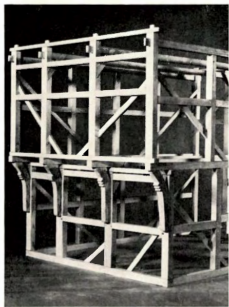
Model af trefagshusets oprindelige tømmerkonstruktion udført af John Kronborg Christensen og Tony Bødtker Munch. I øverste række til venstre ses torvesiden og østgavlen, og til højre østgavlen i front. I nederste række til venstre har vi torvesiden i større mål og til højre østgavl og bagside set sammen. Fot. J. K. C. 1976.
