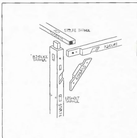
b. Samling mellem stolpe, bjælke og kopbånd samt mellem stolpe og tagrem. Tømmerstykkerne trukket fra hinanden.
