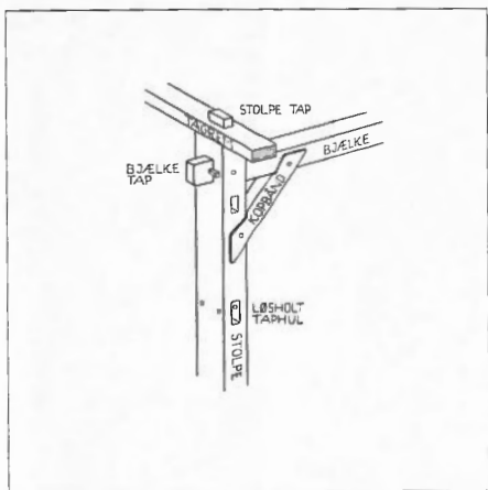
a. Samling mellem stolpe, bjælke og kopbånd samt mellem stolpe og tagrem. Skråprojektion gengivet i mål 1:50.
