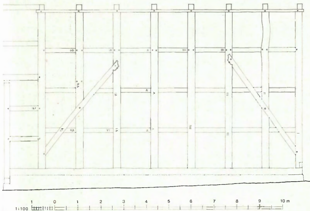
Høxter (v. Hildesheim), Westerbach Str. 34. Ottefags gavlhus med to udvendige ranker i langsiderne. Rankerne er forneden tappede i stolperne og foroven fastgjort med hageblad. Bygningen bærer årstallet 1537. Gengivet i målestok: 1:100. Opmålt af HHE 1970. (A.B.).
