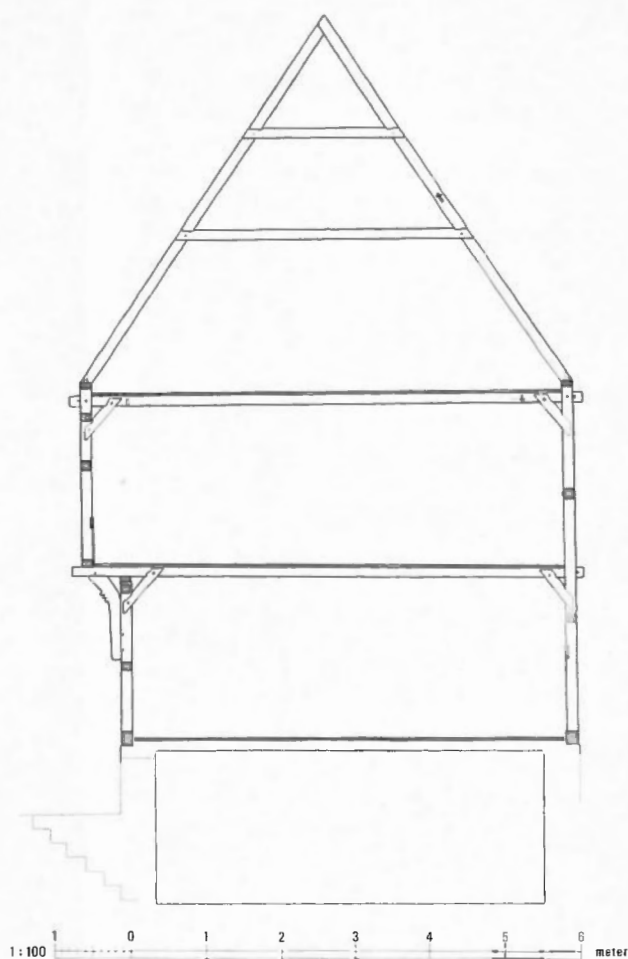
Tværsnit i trefagshusets 1. fag – set mod vest, rekonstruktion.
