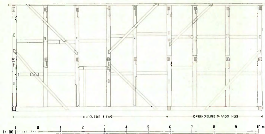
Rekonstruktion af bagsiden set indefra, tegnet på grundlag af C. A. Jensens skitseopmåling fra 1914, suppleret med iagttagelser gjort under bygningsundersøgelserne i 1975. Signaturer: Eksisterende i 1914 – tyk streg. Sikker rekonstruktion – tynd streg. Usikker rekonstruktion – prikket.
