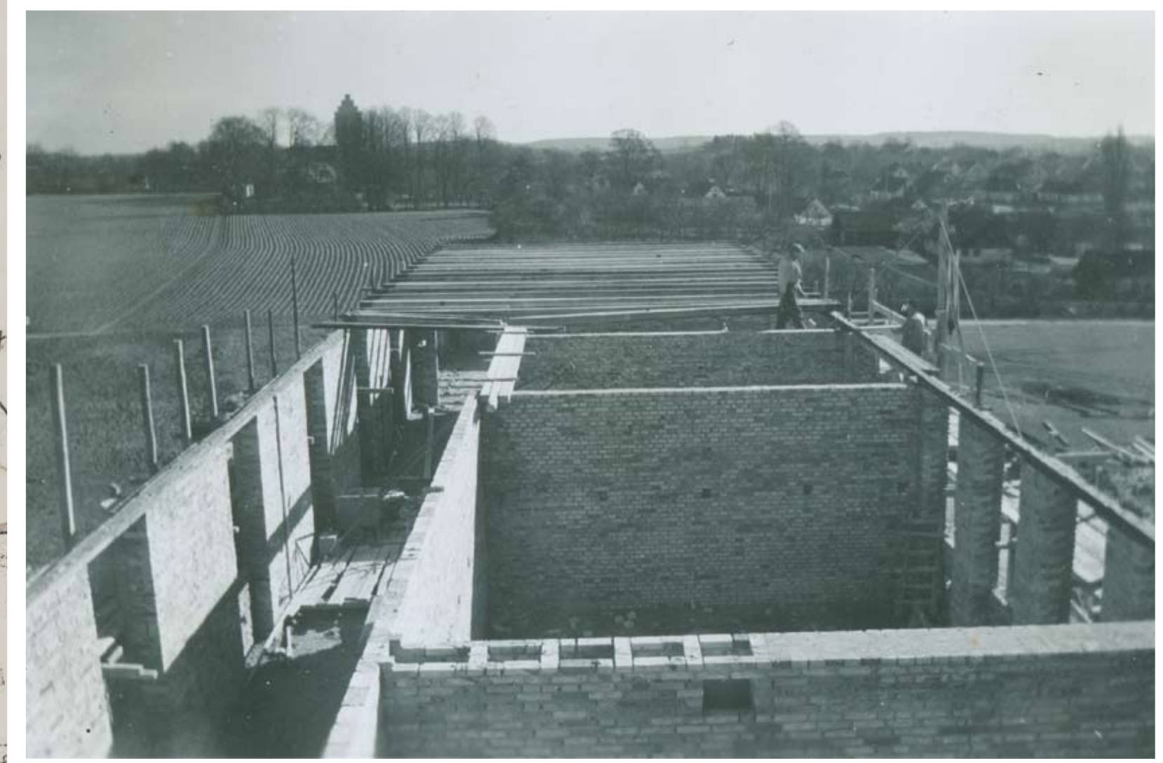
Bjælkelaget lægges ud.
