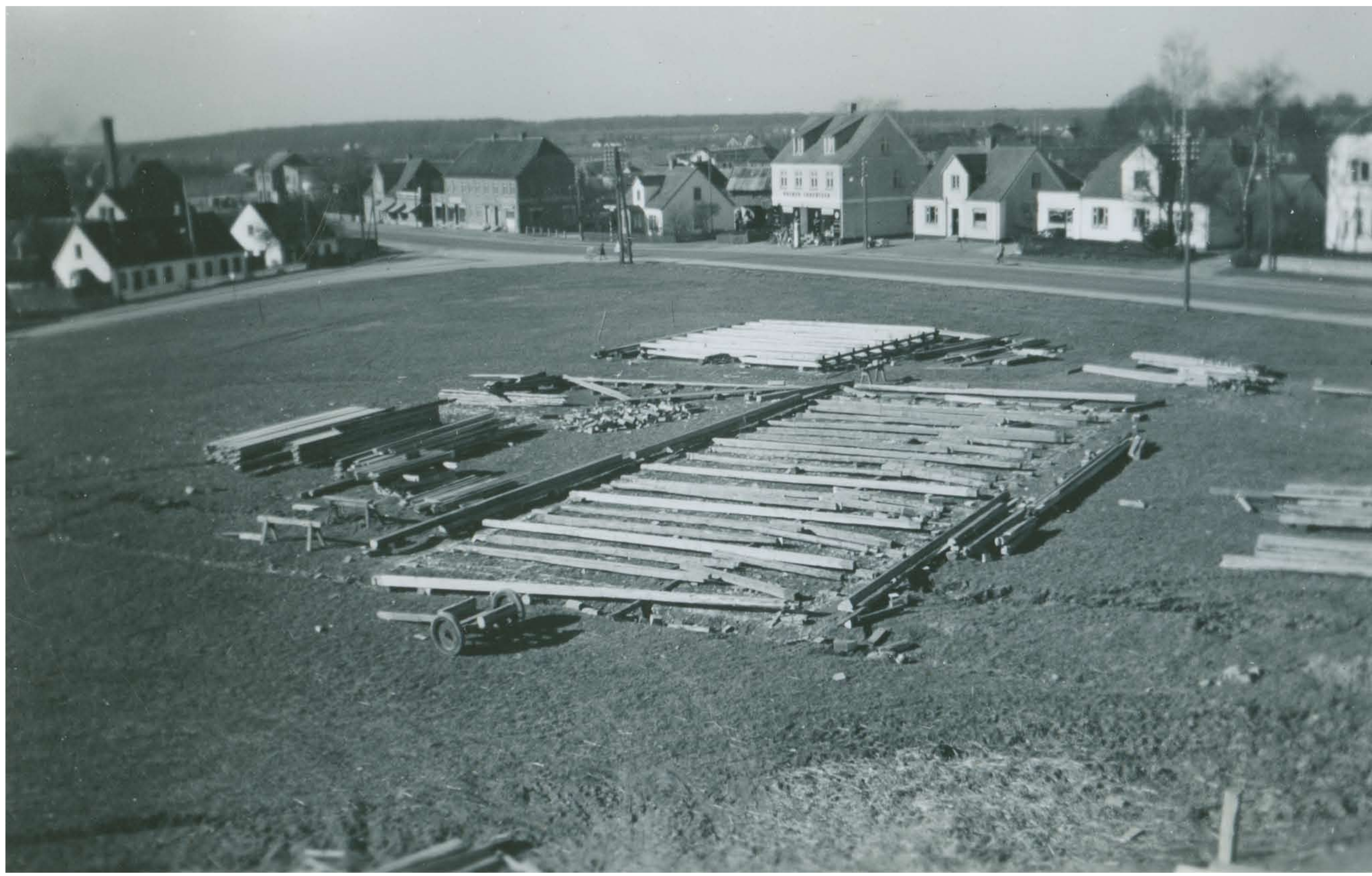
Spærtræ klar til rejsning på afbindingspladsen. Bemærk Vordingborgvej i baggrunden.
