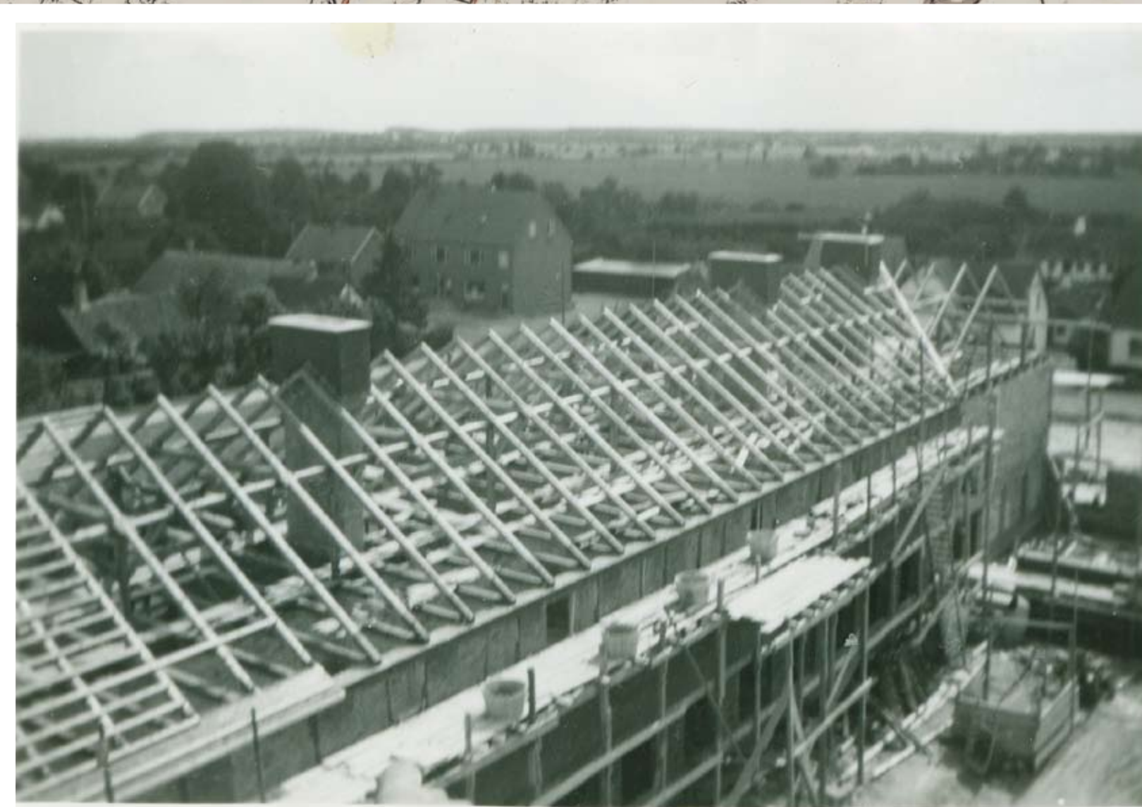
Østfløjens tagkonstruktion.
